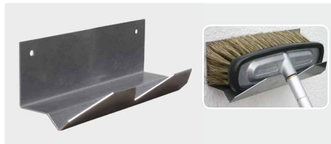
Geeignet für alle Bürsten. Lochabstand 202 mm. H x B x T = 90 x 250 x 100 mm
