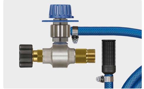
M22 IG : M22 AG. Injektor mit Dosierventil ST-161, Saugschlauch 2.000 mm und Saugfilter ST-31. Max. 350 bar / 90 °C
