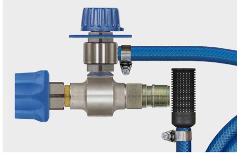
Kupplung ST-45-250 Messing vernickelt : Stecknippel ST-45-250 Stahl verzinkt. Injektor mit Dosierventil ST-161, Saugschlauch 2.000 mm und Saugfilter ST-31. Max. 250 bar / 90 °C
