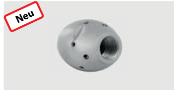
3/8" IG. 6x 75° 3x 30° +1x 0°. 30-100 l/min. Für \text{R} \text{D} 100-200 mm. Außen \text{D} 35 mm. \text{G} 314 g.
