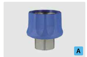
Kupplung : IG. Messing vernickelt. Max. 250 bar / 150 °C
