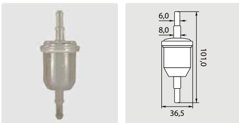
Leitungsölfilter
