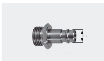
Stecknippel : AG. Edelstahl. Max. 150 bar / 90 °C
