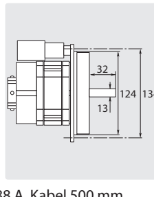
Flansch und Pumpenaufnahme 32 mm
