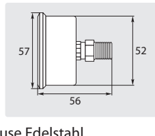
∅ 50 mm. 1/4" AG. Gehäuse Edelstahl. Eingang hinten
