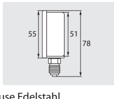
∅ 50 mm. 1/4" AG. Gehäuse Edelstahl. Eingang unten
